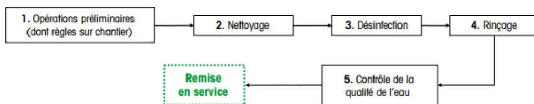
Figure 4 : Procédure complète de nettoyage et de désinfection d'une canalisation d'eau destinée à la consommation humaine (santé.gouv.fr)
