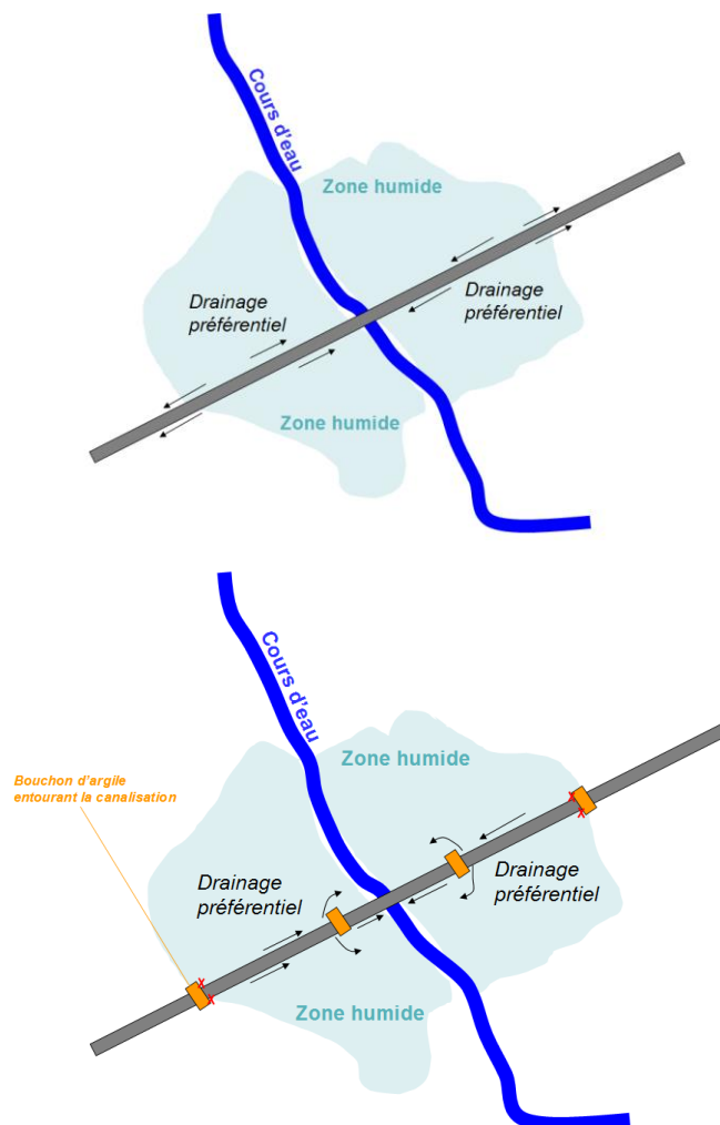
Figure 1 : Principe de mise en place d'écrans d'argile et effets : sans écrans (1ère figure), avec écrans (2ème figure)
