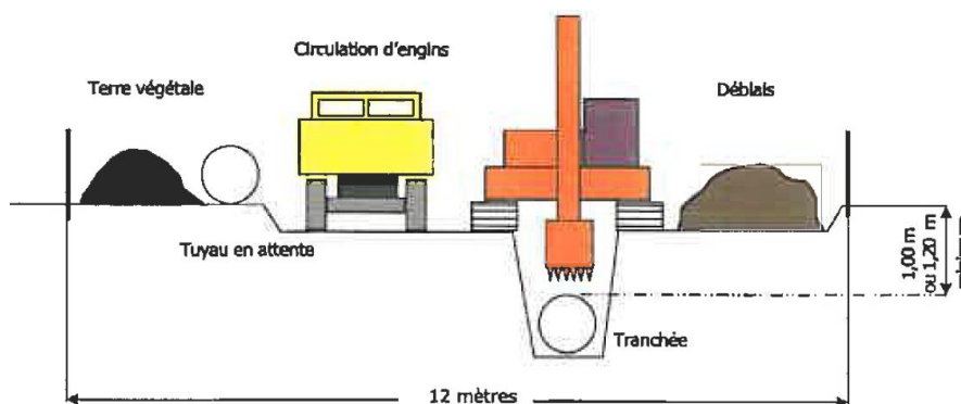
Figure 2 : Profil en travers type de la zone de travail (emprise réduite à 8 mètres en zones humides)
