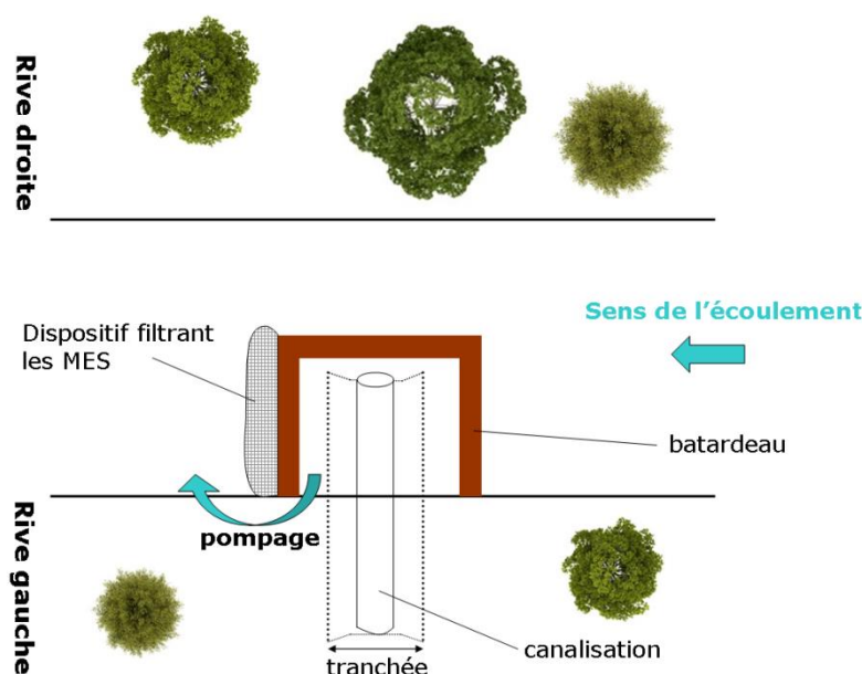
Figure 3 : Schéma détaillant les travaux par demi-section de cours d'eau
